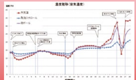
2017/4/3 新潟→マレーシア 輸送試験 温度変化のグラフ
